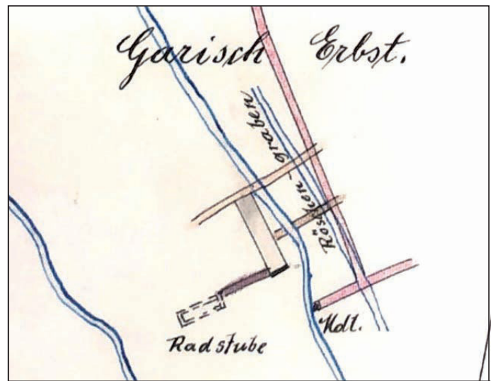
Dieser 1915 gezeichnete Riss zeigt die Lage der Radstube mit der Verbindung zum vermutlich „neuen Kunstschaft“.
